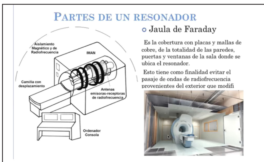
Figura No. 6: Partes de un resonador.
