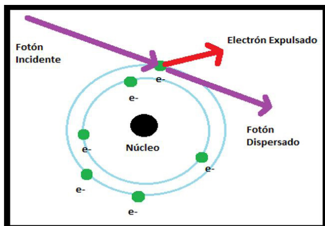
Figura 1: Efecto Compton.
