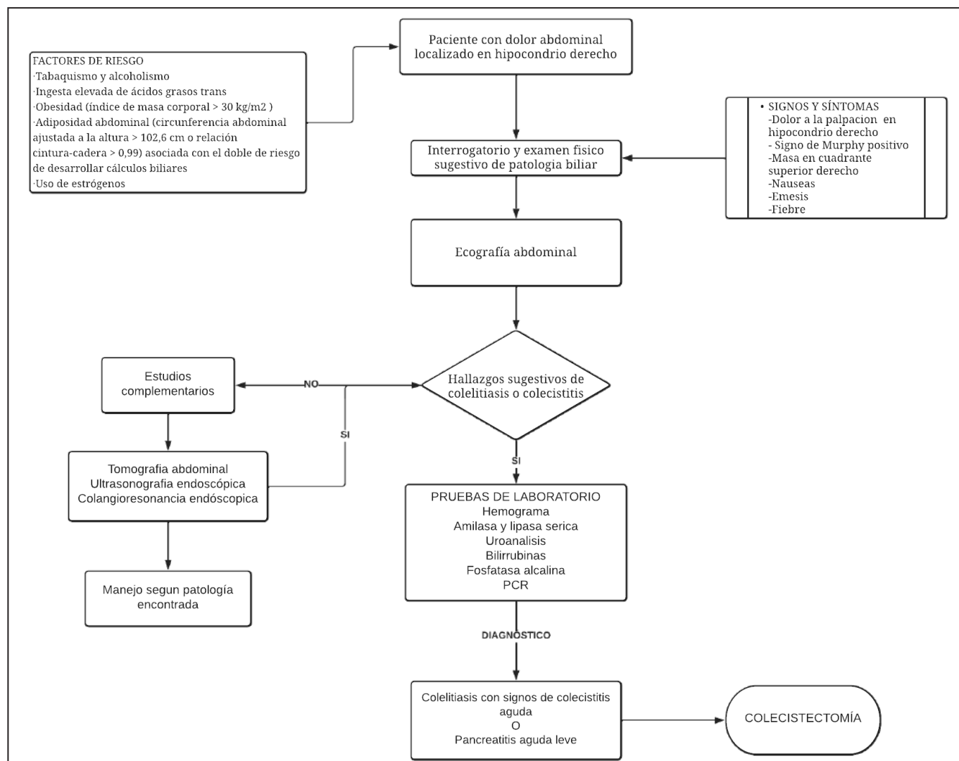
Figura 6: Algoritmo diagnóstico.
